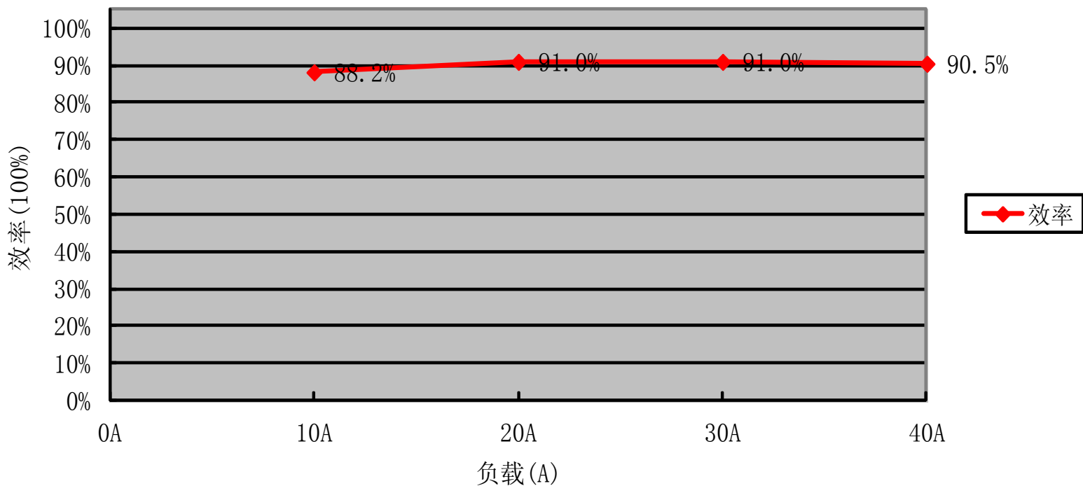
负载与效率曲线
