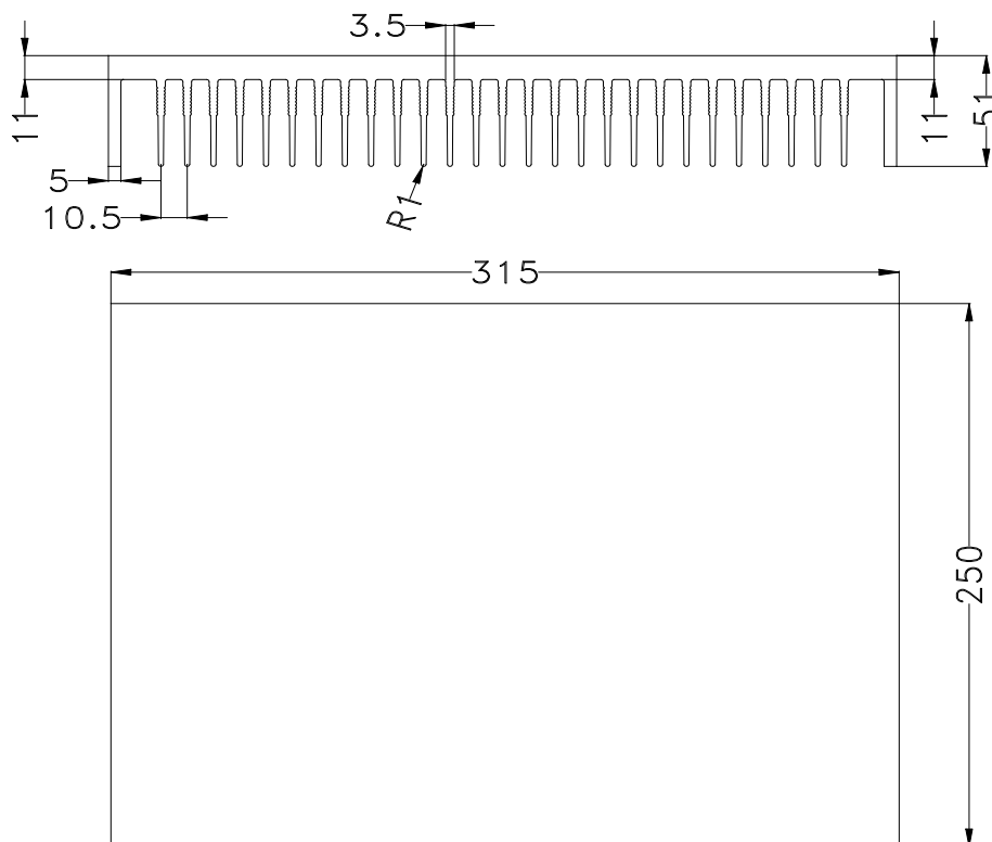
图一 Scheme for Heatsink 散热板尺寸图
